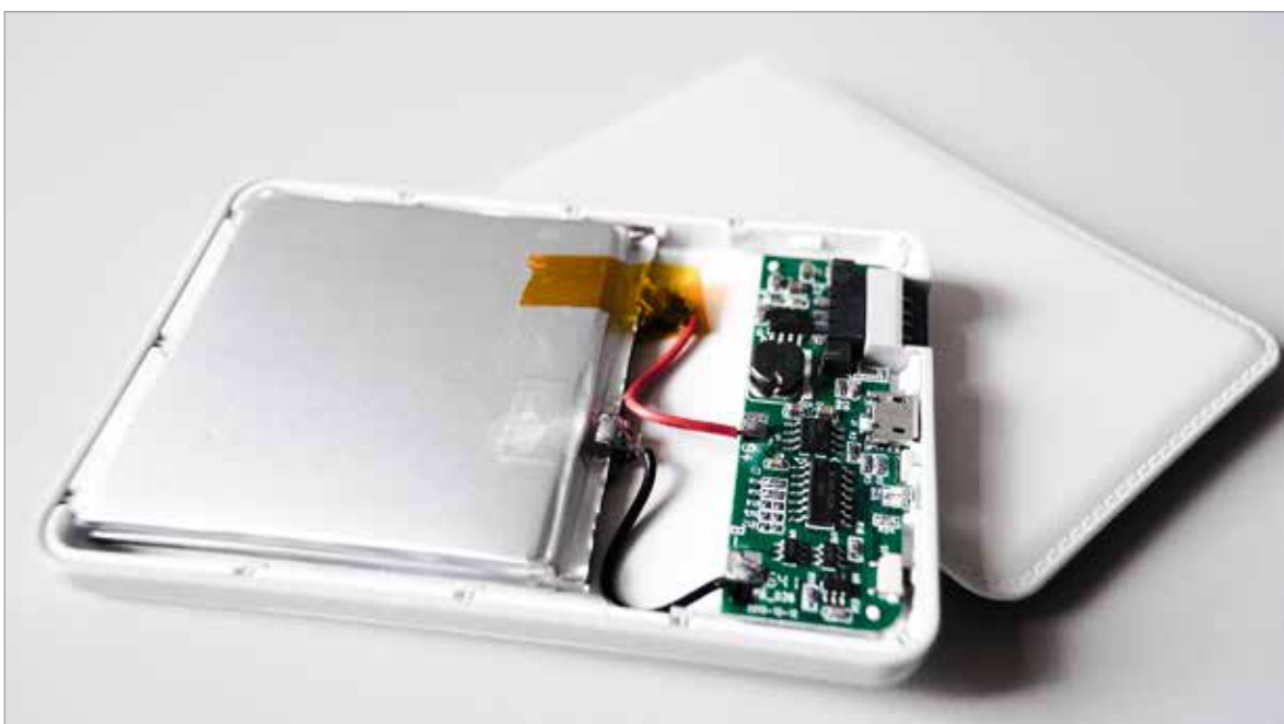
Abb. 12: Pouch-Lithium-Ionen-Zelle mit einer Kapazität von 4.000 mA (BGR 2017).
