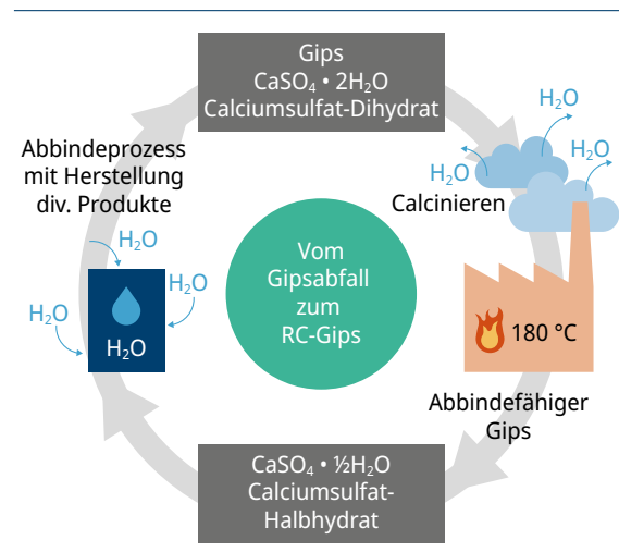
Abb. 25: Vom Gipsabfall zum RC-Gips (BV Gips 2023)
