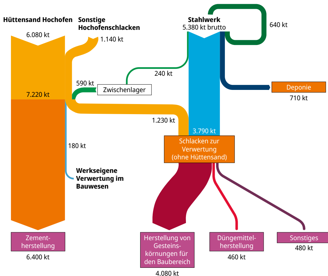
Abb. 22: Stoffströme der Schlacken und Hüttensande aus der Eisen- und Stahlerzeugung in Deutschland 2015 (UBA 2019b)
