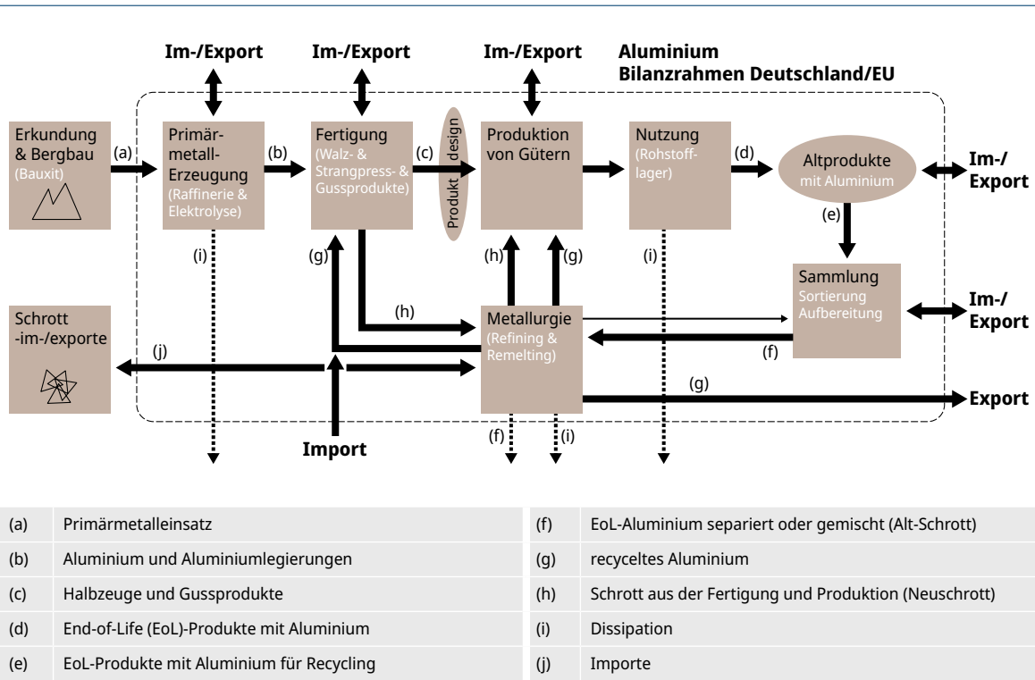
Abb. 7: Referenzgrafik Stoffstrom Aluminium in Anlehnung an UNEP (2011)
